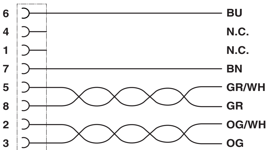
Diagrama eléctrico
