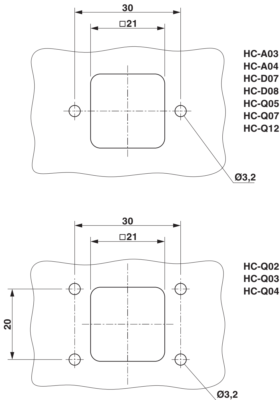
Dessin coté
