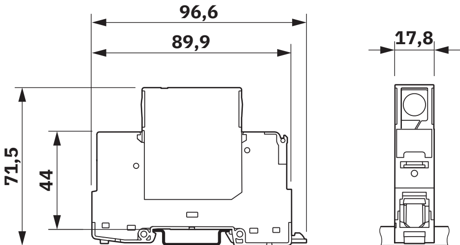
Maßzeichnung
