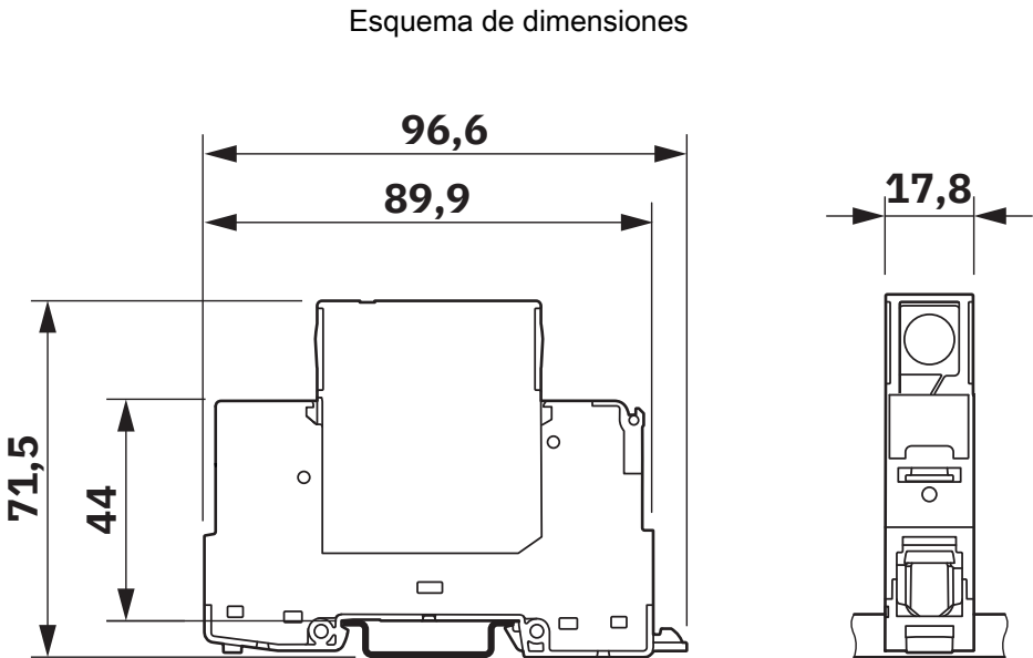
Plano esquemático
