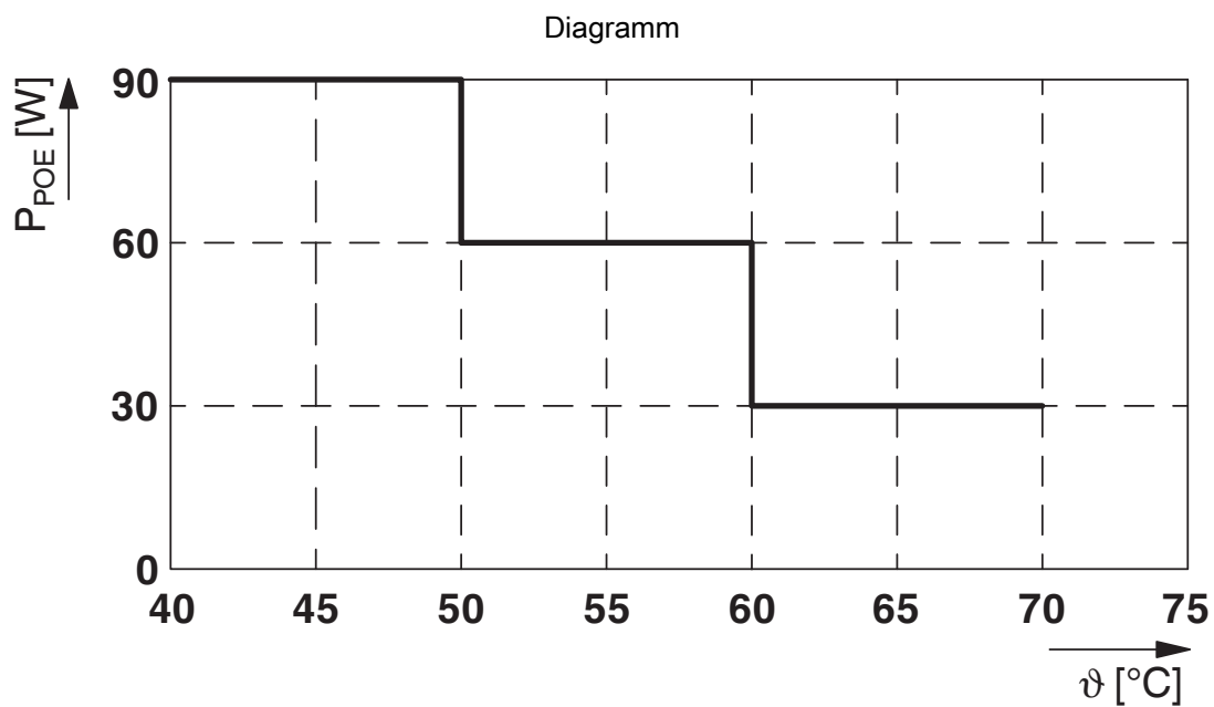
Derating (PoE-Leistung gesamt)
