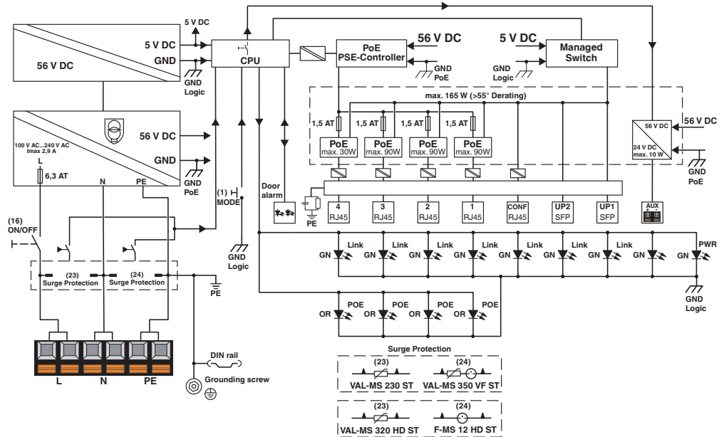
Diagrama eléctrico
