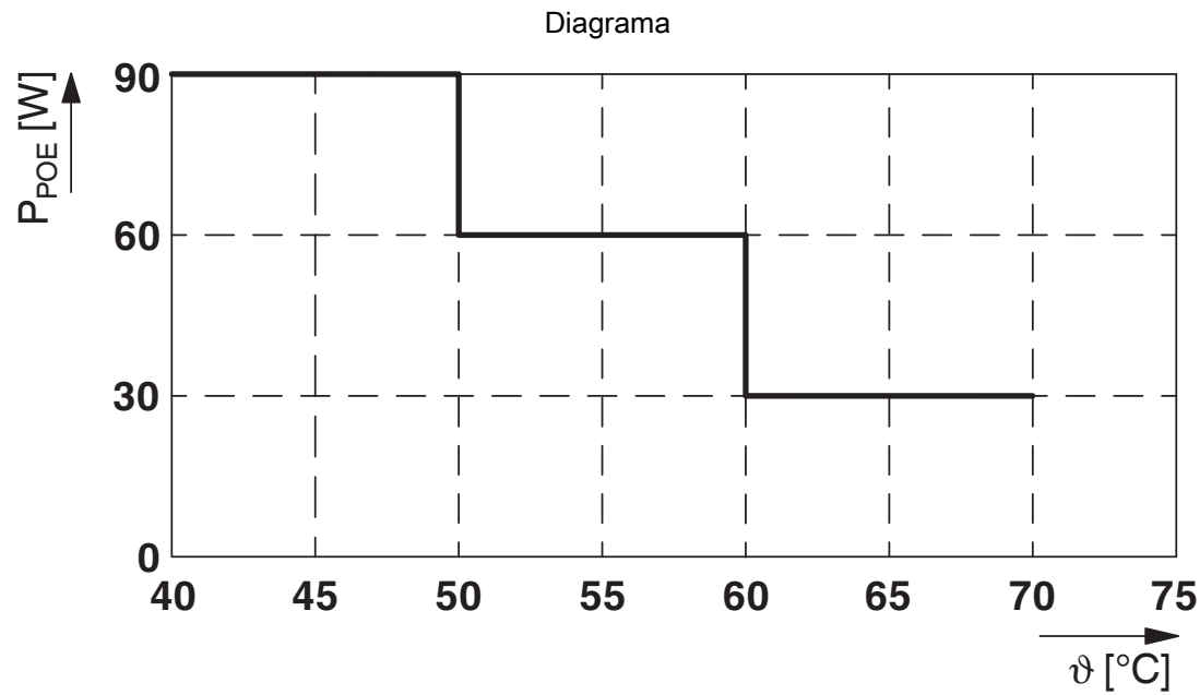
Derating (potencia PoE total)
