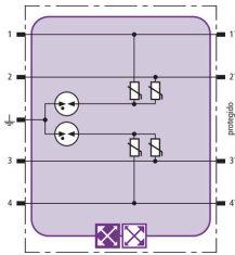
Esquema del BXT ML4 MY 110
