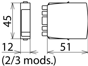
Dimensiones del BXT ML4 MY 110
