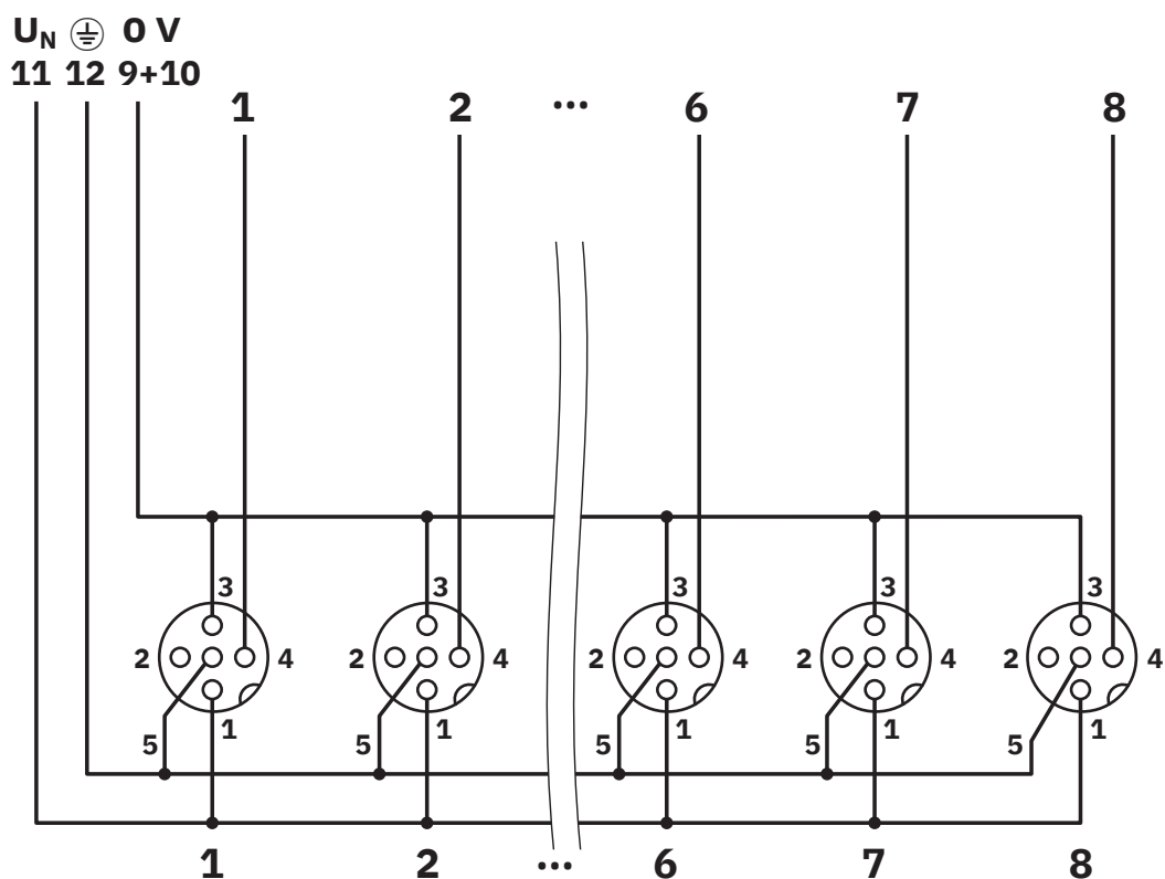
Diagrama eléctrico
