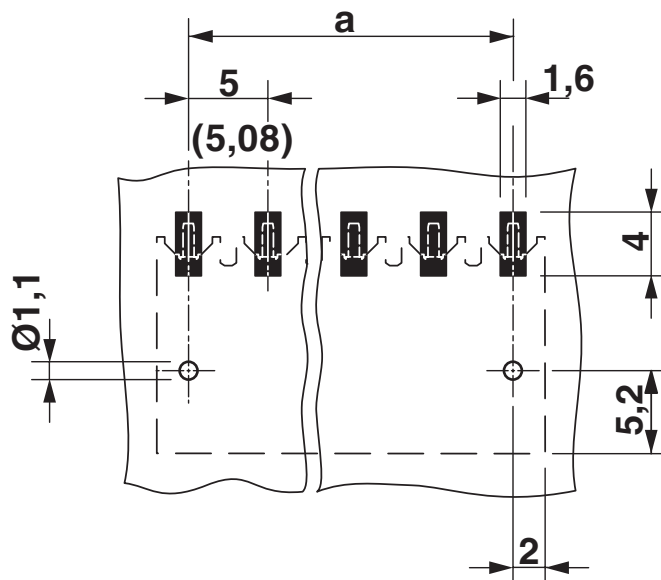
Bohrplan/Lötpadgeometrie
