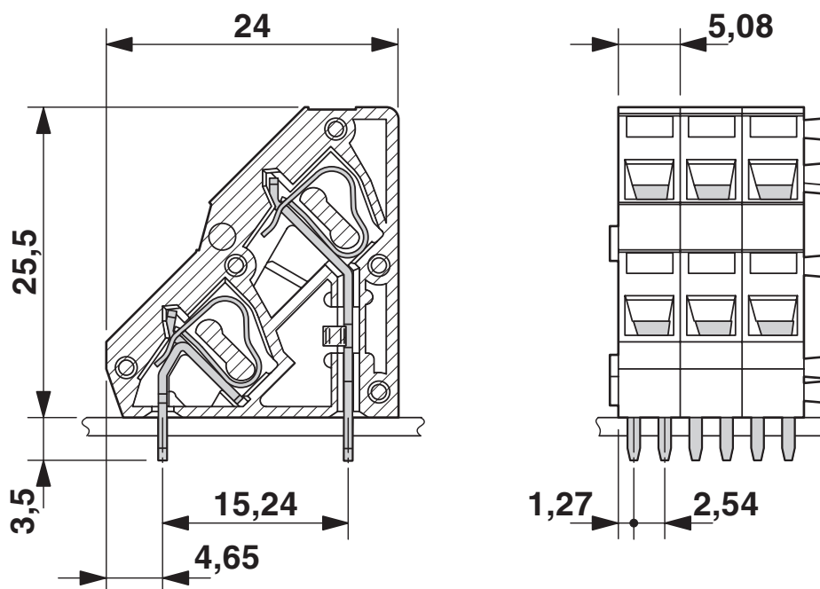
Maßzeichnung
