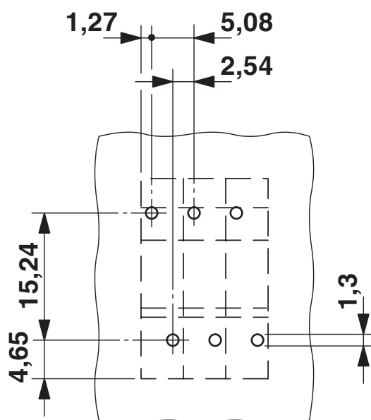
Bohrplan/Lötpadgeometrie
