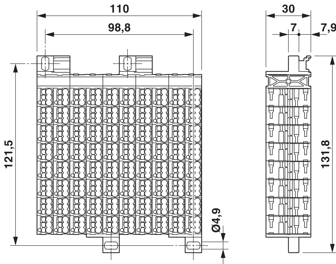
Dessin coté
