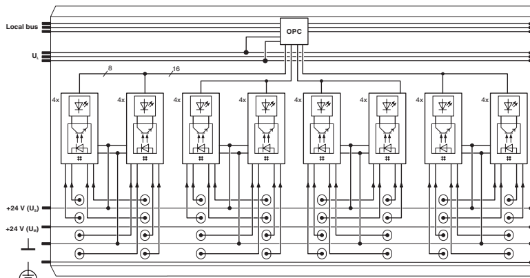
Schéma fonctionnel
