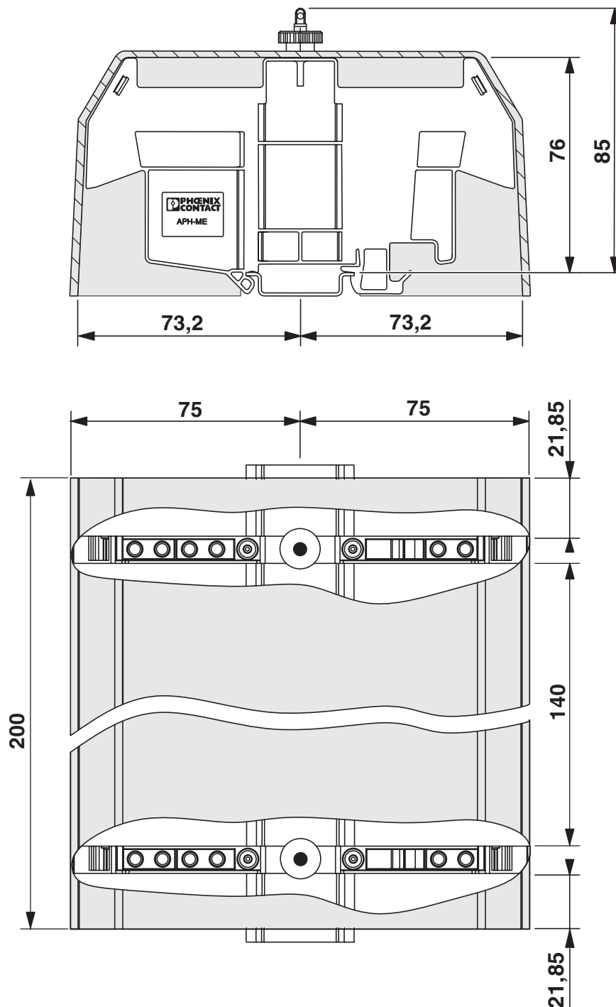
Dessin coté
