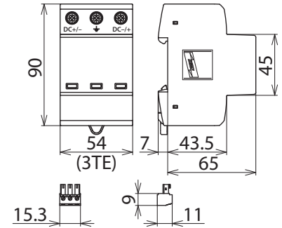
Maßbild DG YPV SCI 1000 FM
