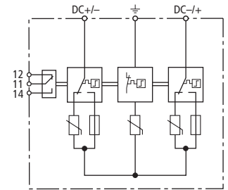
Prinzipialschaltbild DG YPV SCI 1000 FM
