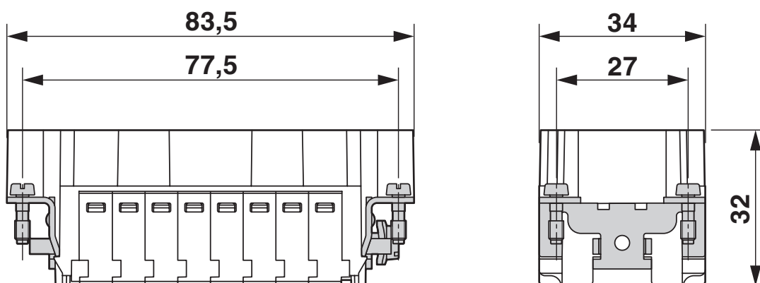
Maßzeichnung
