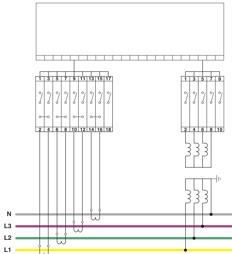
Diagrama eléctrico
