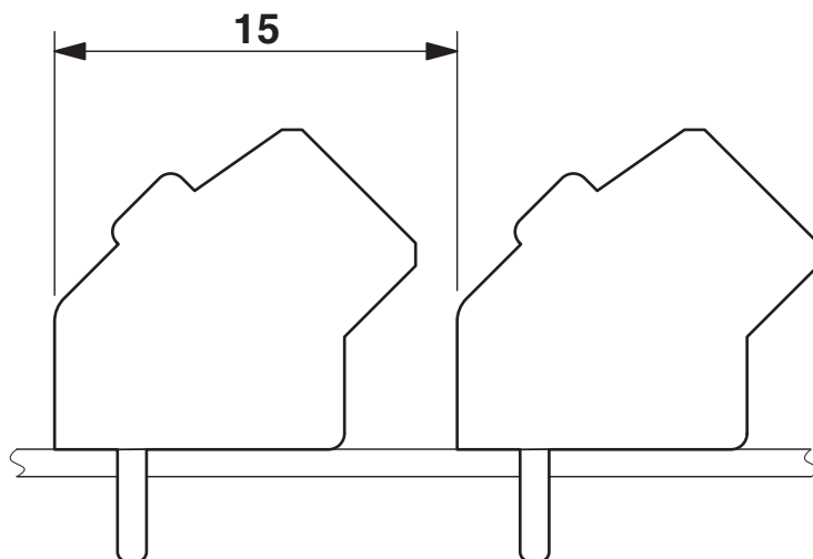
Dessin coté
