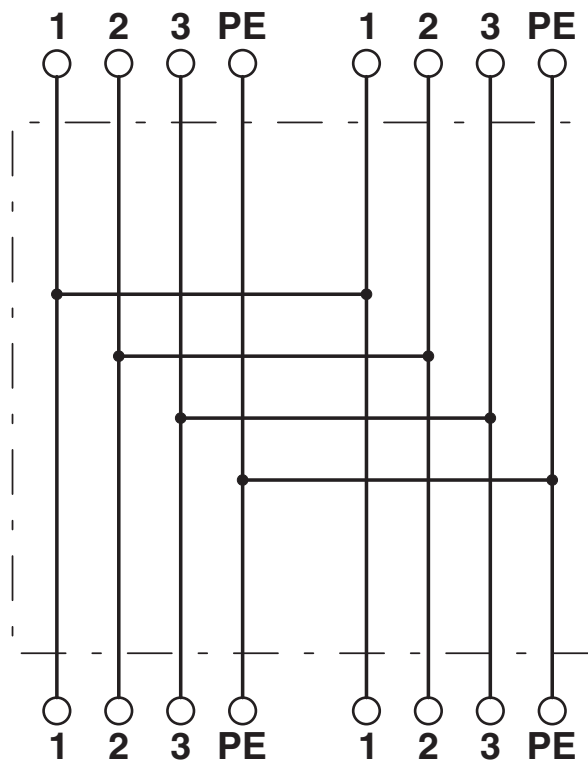
Diagrama eléctrico
