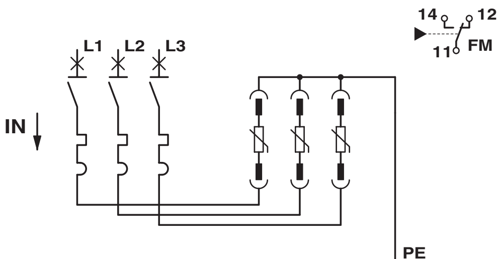
Diagrama eléctrico
