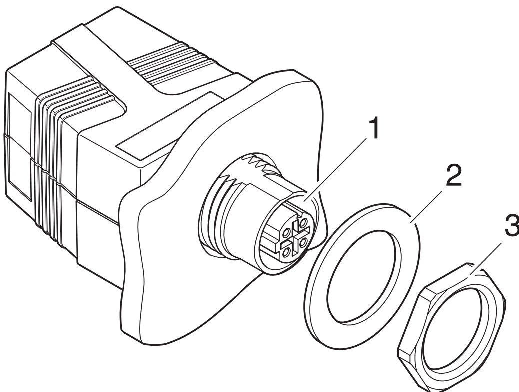
Explosionszeichnung
