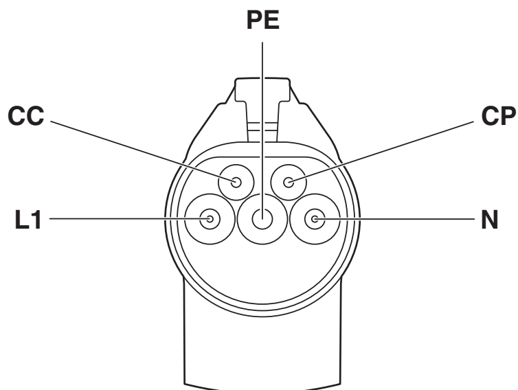
Affectation des broches connecteur de charge de véhicule
