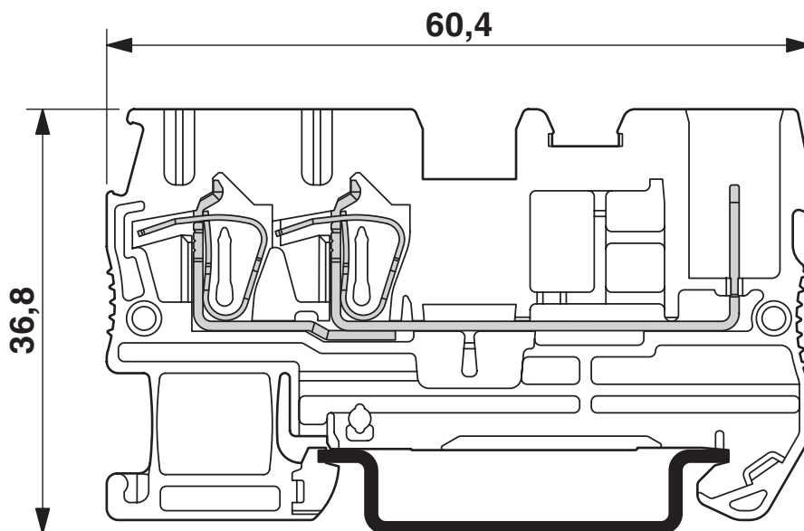
Dessin coté
