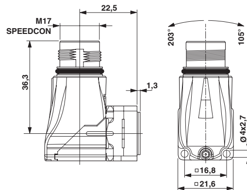
Dessin coté
