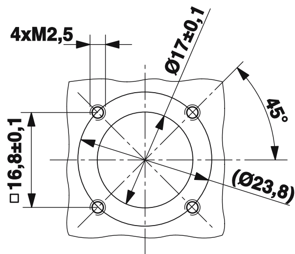
Dessin coté
