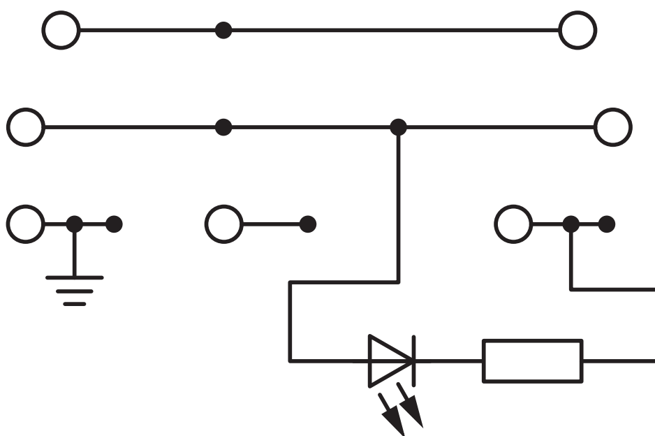
Diagrama eléctrico
