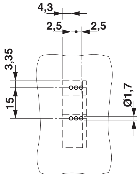
Bohrplan/Lötpadgeometrie
