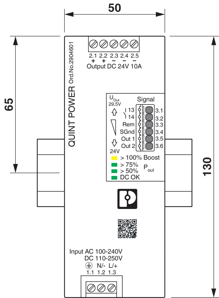
Dessin coté
