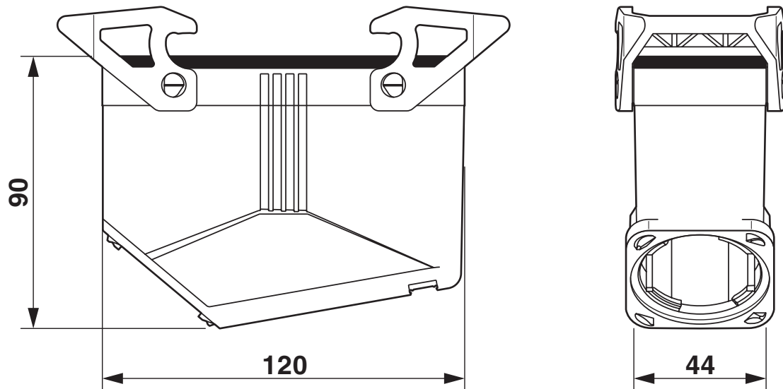
Maßzeichnung
