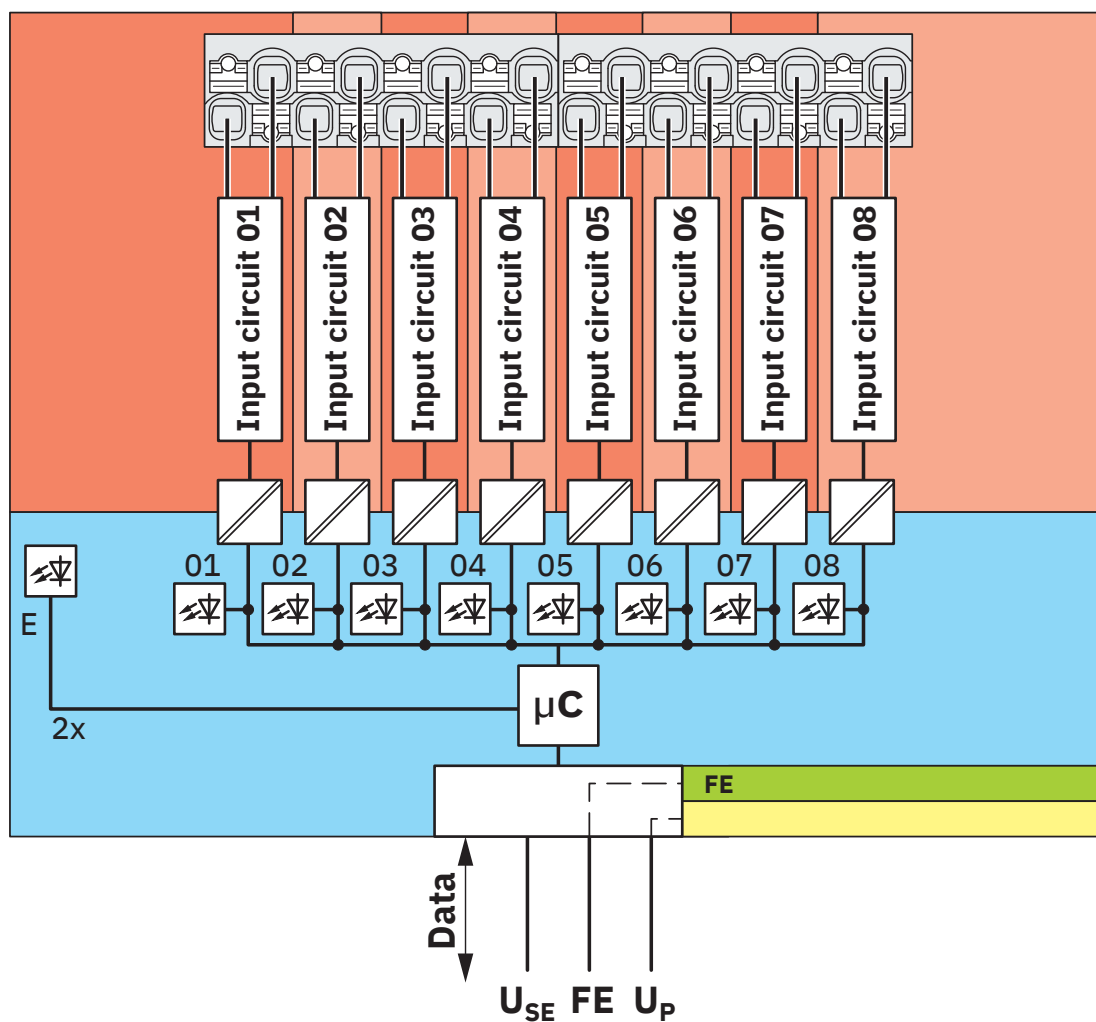
Schéma fonctionnel
