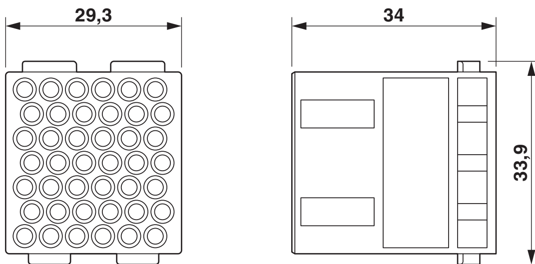
Dessin coté
