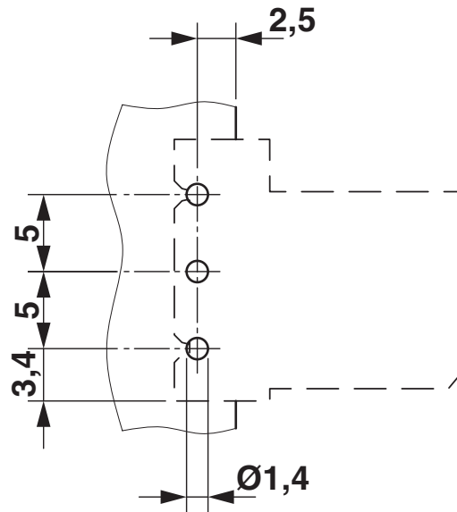
Bohrplan/Lötpadgeometrie
