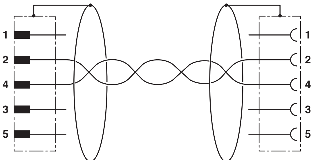
Schaltplan
