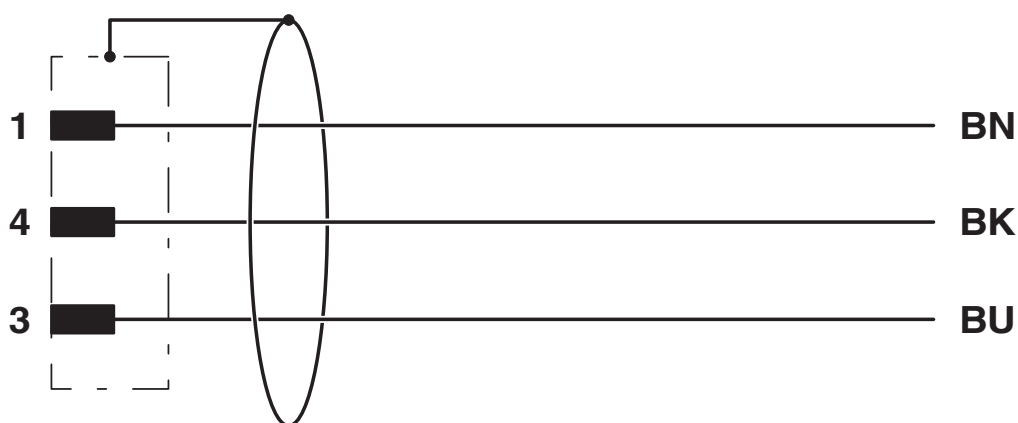
Ocupación de contactos del conector macho M12
