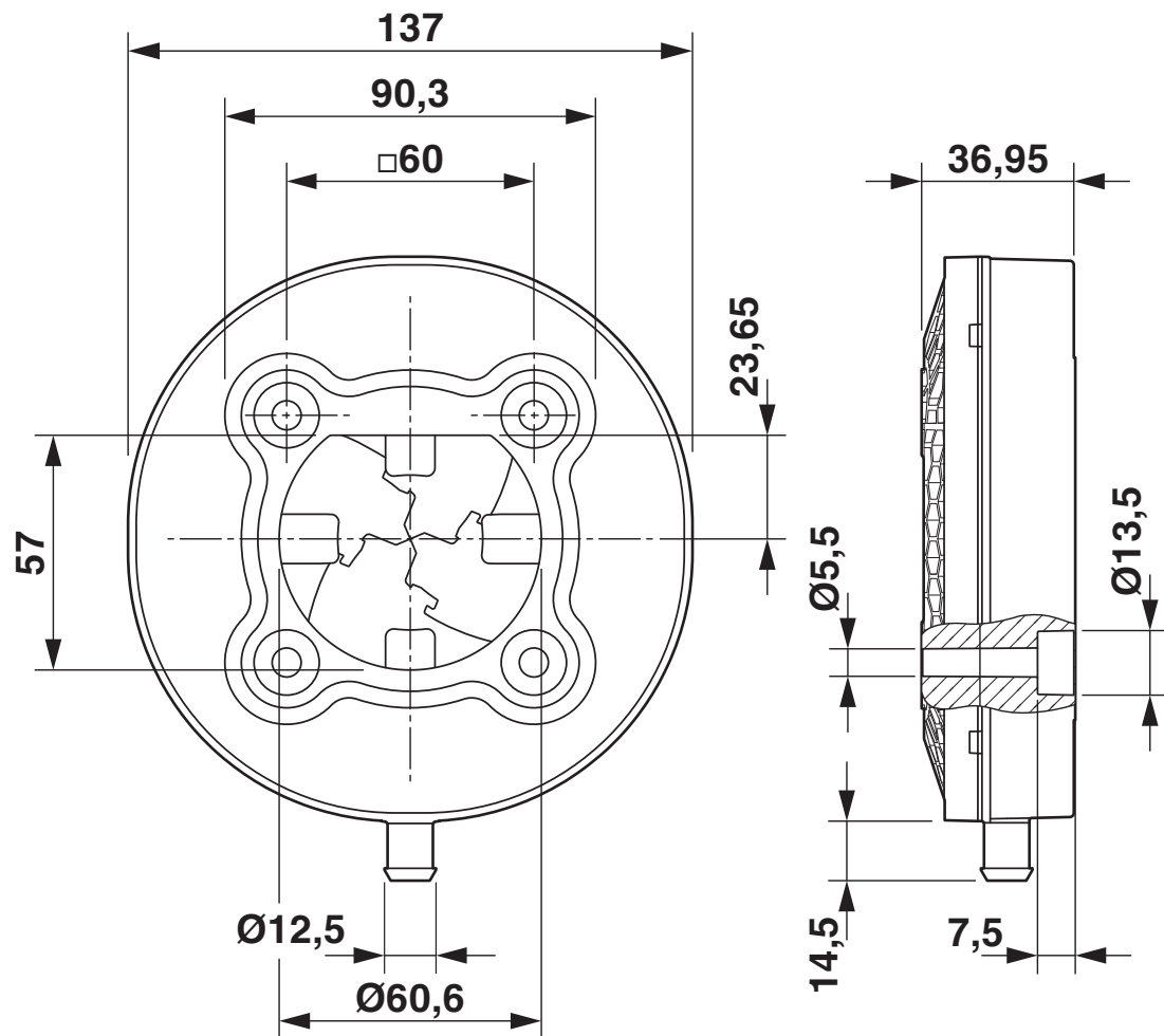
Maßzeichnung
