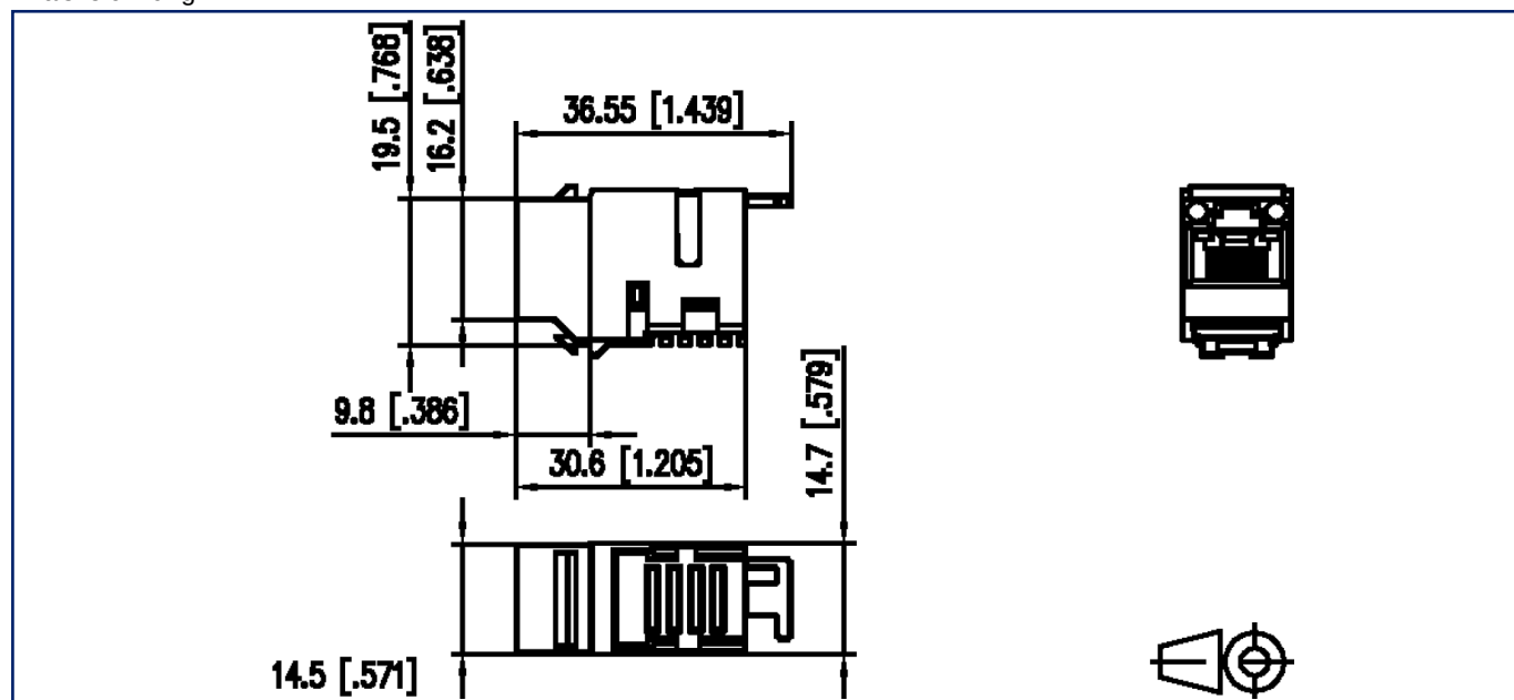
Maßzeichnung
