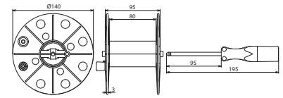
Maßbild DH K 80 BS ML0.75 L100M RT
