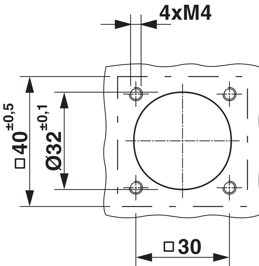
Dessin coté
