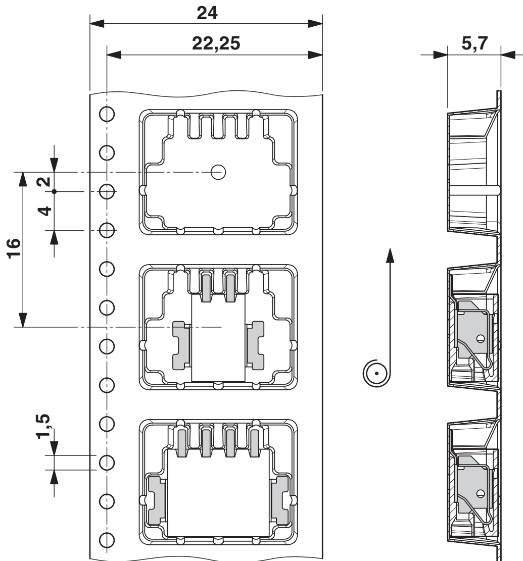
Maßzeichnung
