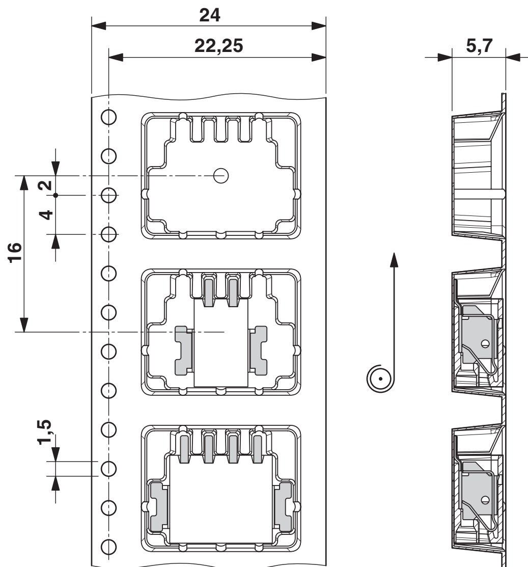
Dessin coté
