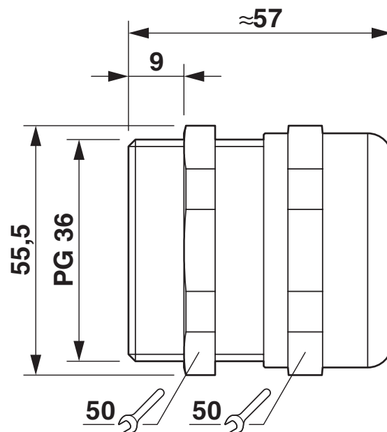
Maßzeichnung
