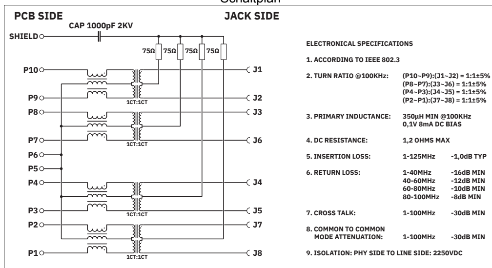
Schaltplan
