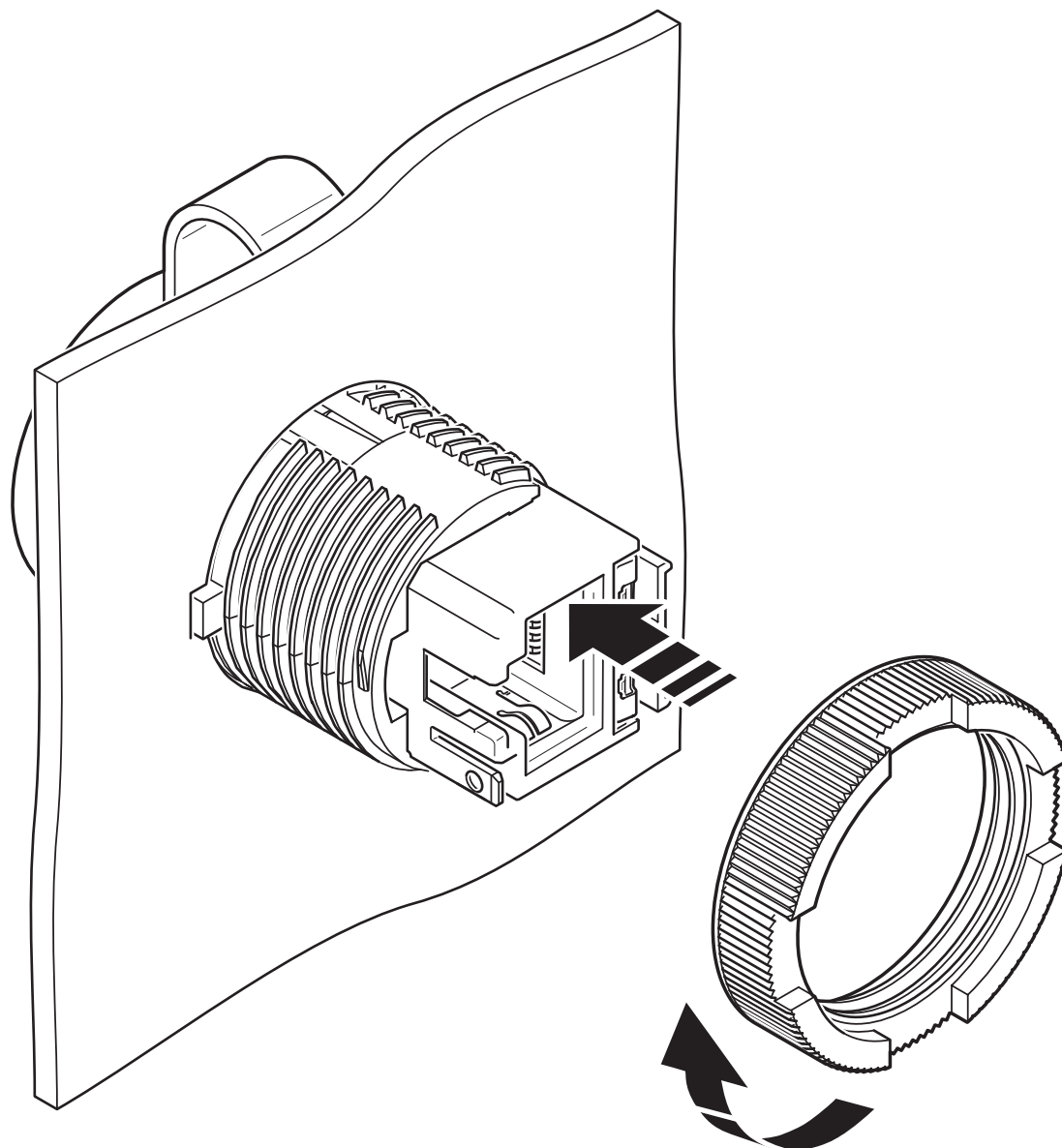
Dessin schématique 2
