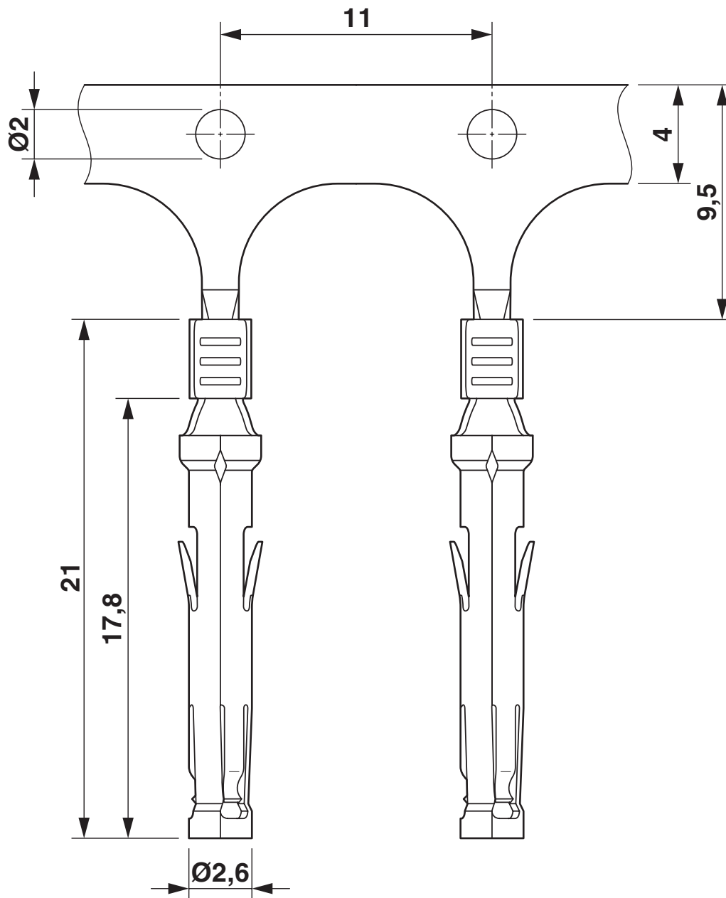
Dessin coté
