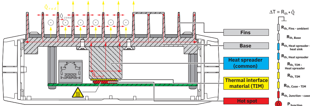
Dessin schématique
