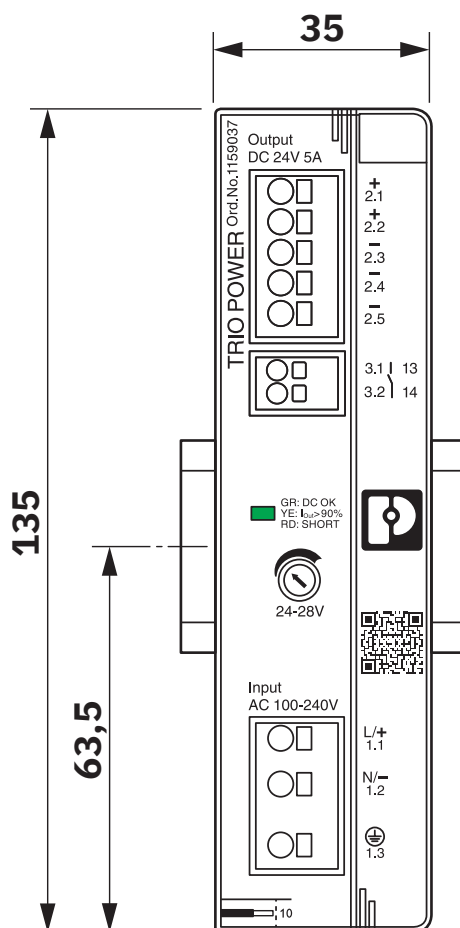
Maßzeichnung
