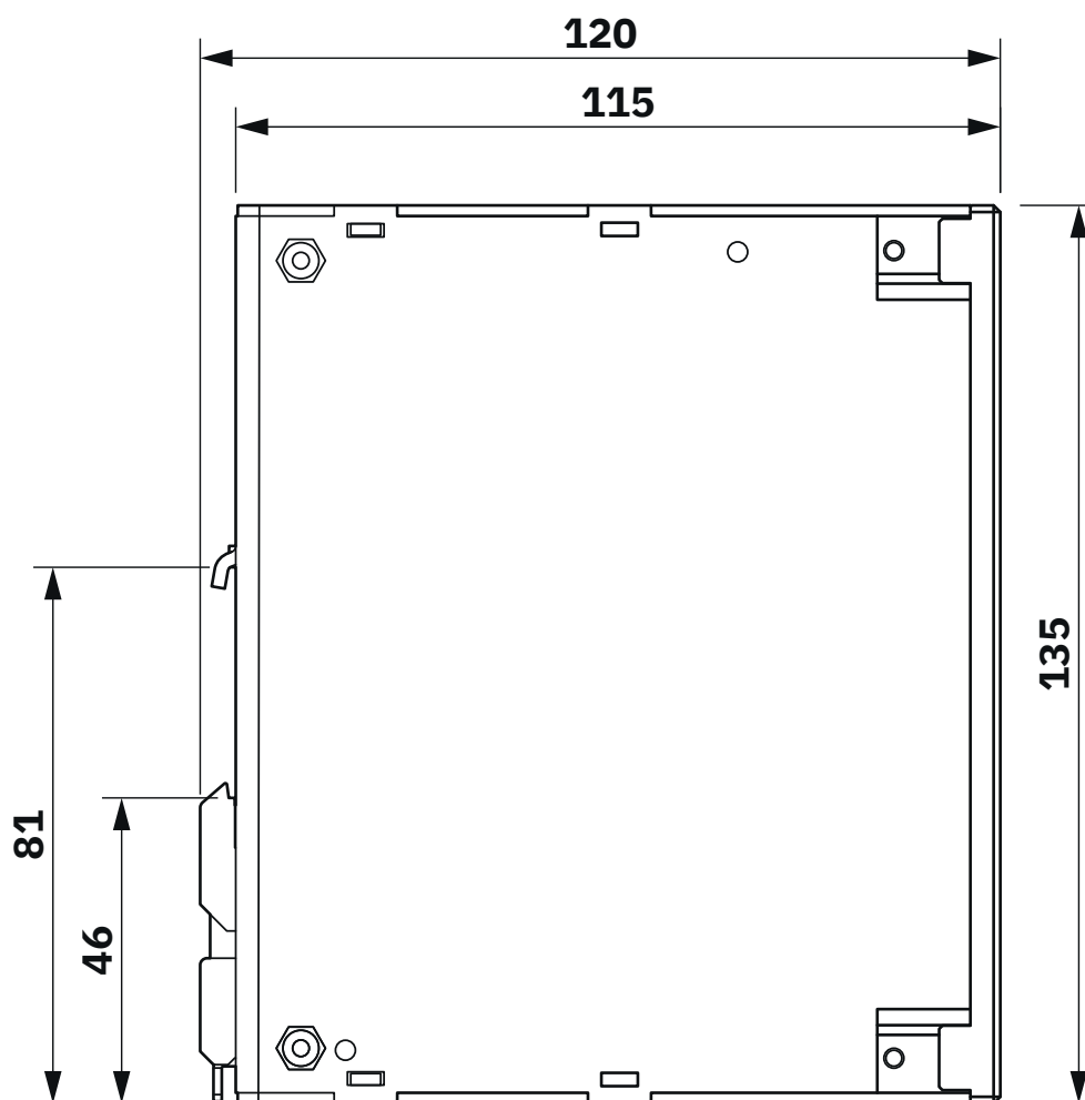
Encombrement de l'appareil (cotes en mm)
