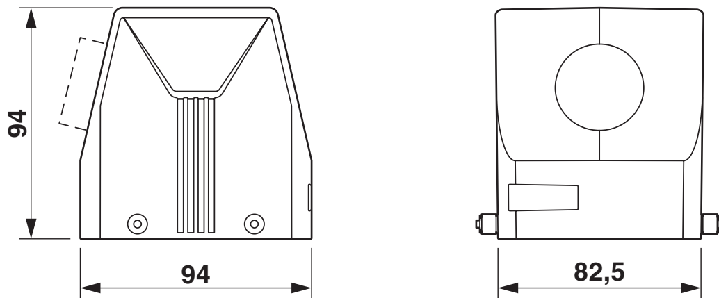
Maßzeichnung
