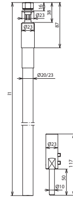
Maßbild HVI RAV 75 23 L6M GR M
