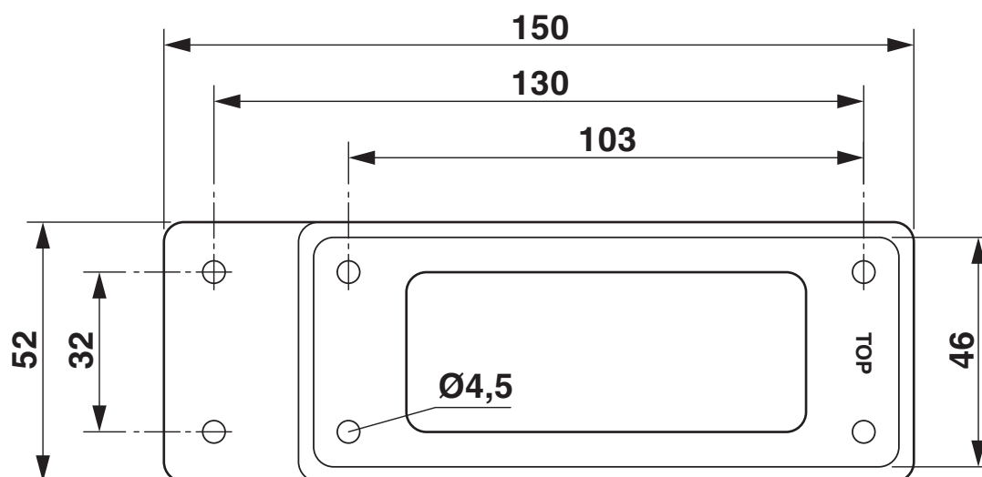
Dessin coté
