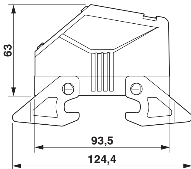
Dessin coté
