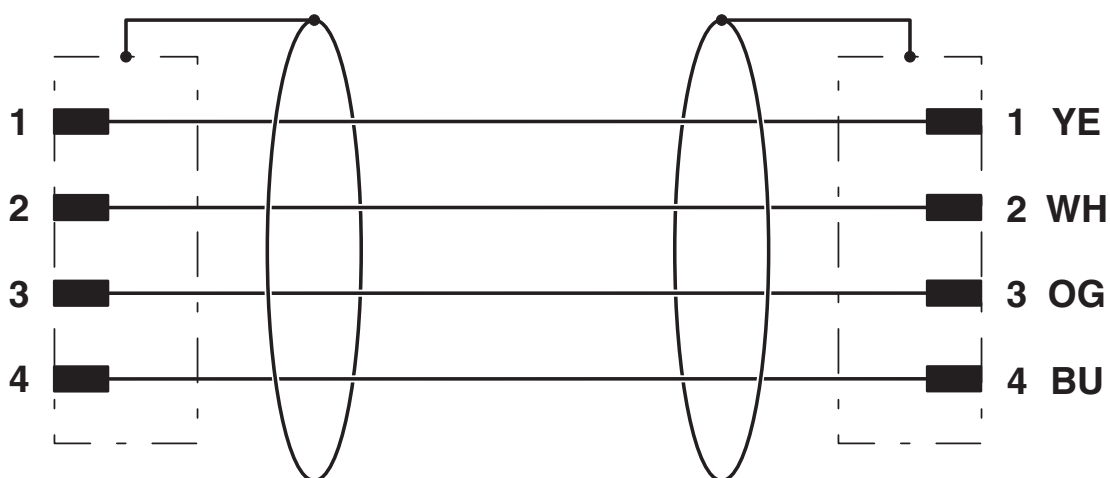
Ocupación de contactos de los machos M12
